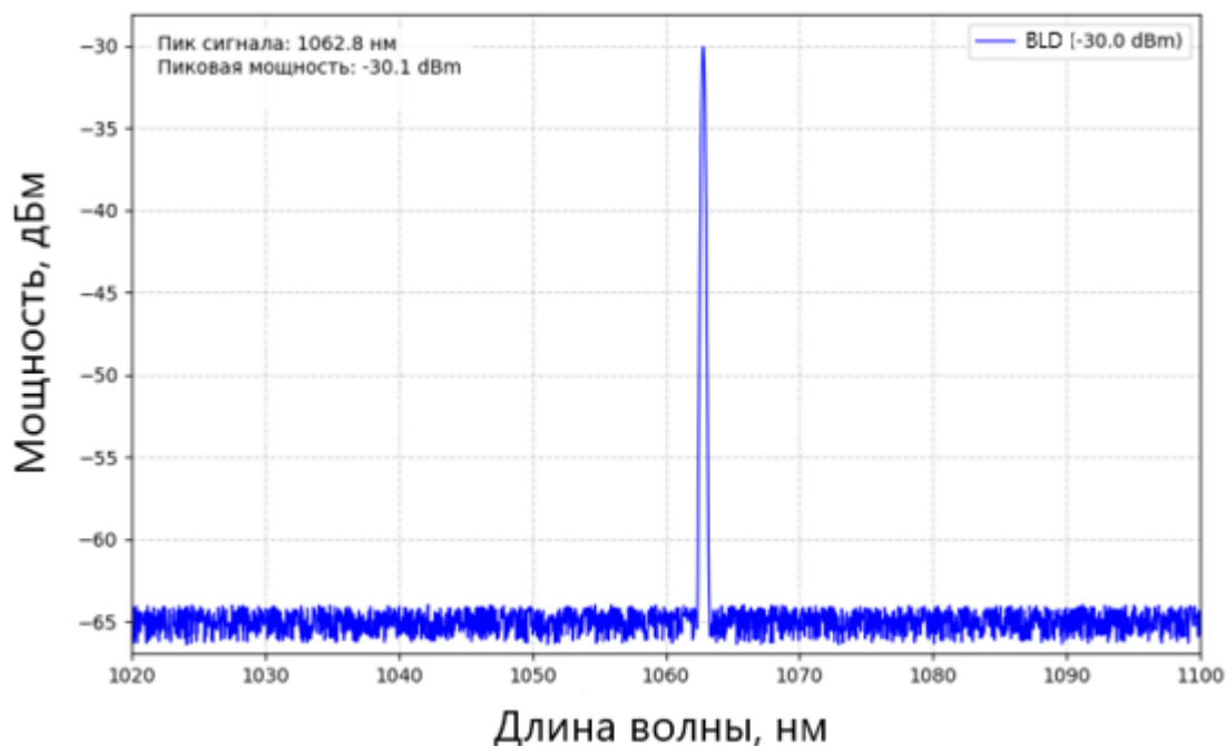
Рисунок 5 – Спектр выходного сигнала BLD лазера
