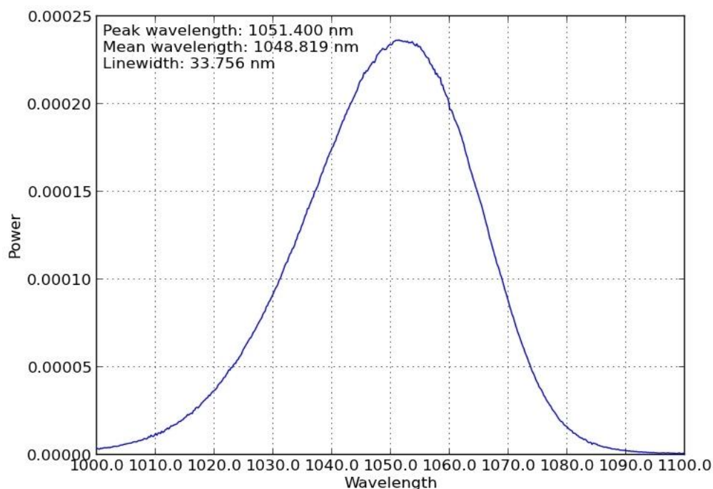
Рисунок 3 – Спектр SOA-1060 при токе накачки 100 мА
