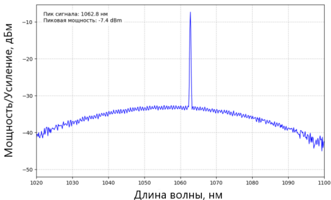
Рисунок 6 – Спектр выходного сигнала BLD лазера с коэффициентом усиления 26–27 дБ
