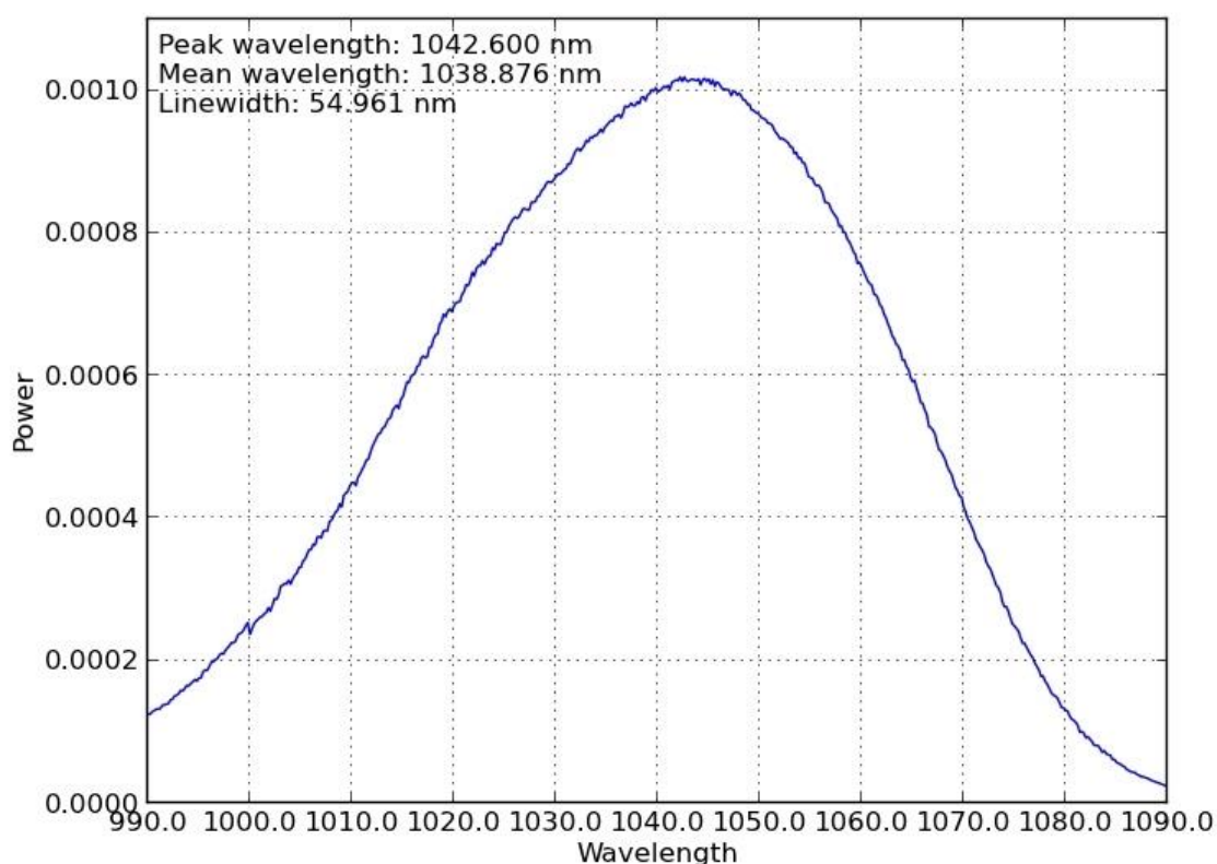
Рисунок 2 – График спектра SOA – 1064 при рабочем токе накачки 300 мА для примера
