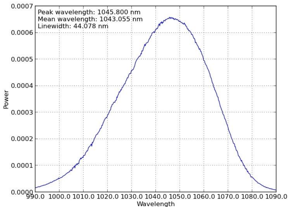
Рисунок 4 – Спектр SOA-1060 при токе накачки 200 мА
