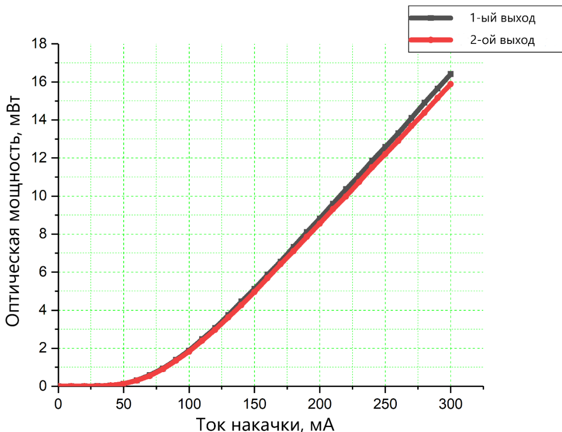
Рисунок 3 – Пример ВТАХ характеристики SOA-1060 в корпусе «14BF» с SM волокном
